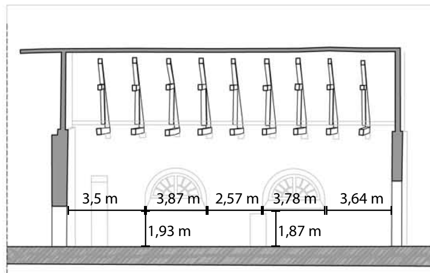
LONG SECTION B-B'
