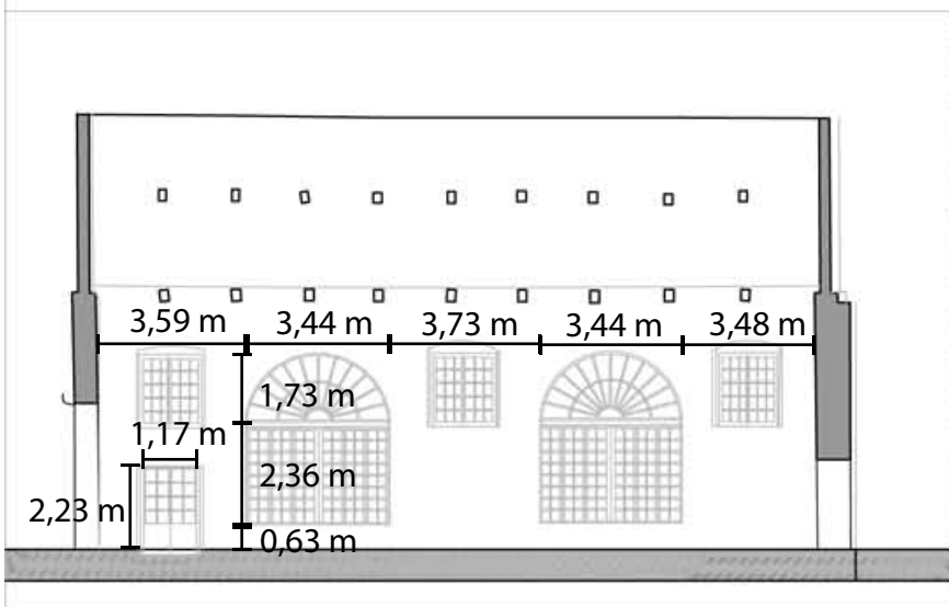
LONG SECTION A-A'
